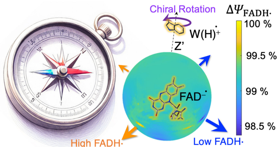
クリプトクロムのキラリティスピン選択性(CISS)による磁気コンパス
