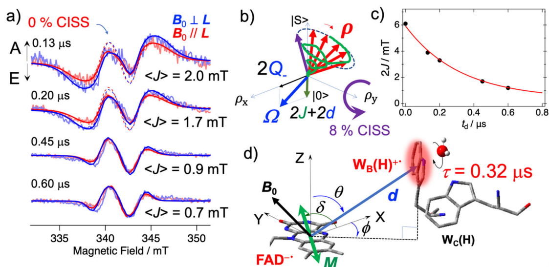
図 1. 時間分解電子スピン共鳴による計測結果 ( -153\text{ }^{\circ}\text{C} ) と、量子論モデルによる光電荷分離構造変化の解析
