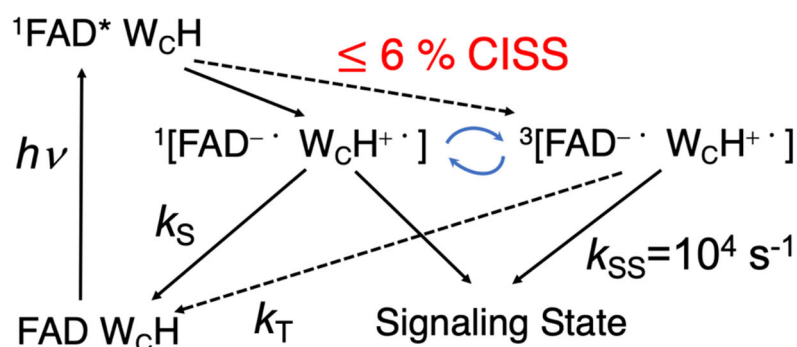
図 2. キラリティスピン選択に伴う、一重項、三重項電荷分離状態のスピン変換と化学反応によるシグナリング反応スキーム
