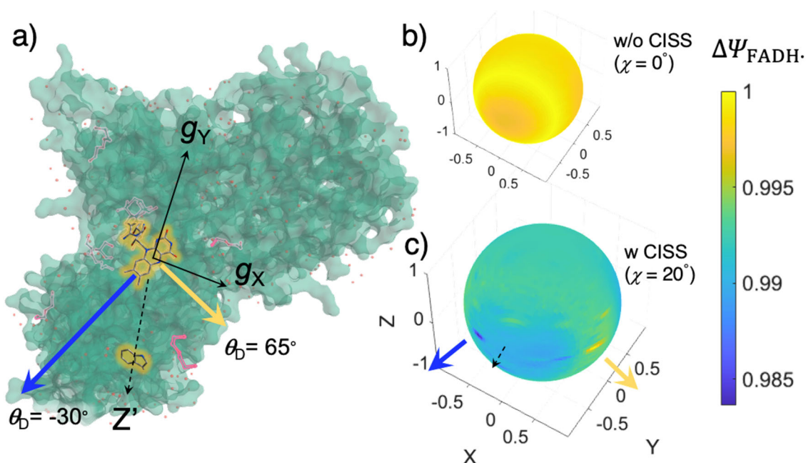
図 3. わずかな CISS 効果が生み出す、シグナリング反応生成収量異方性の増強と磁場方向志向性
